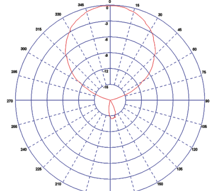
Typisches Vertikales Diagramm 410MHz
